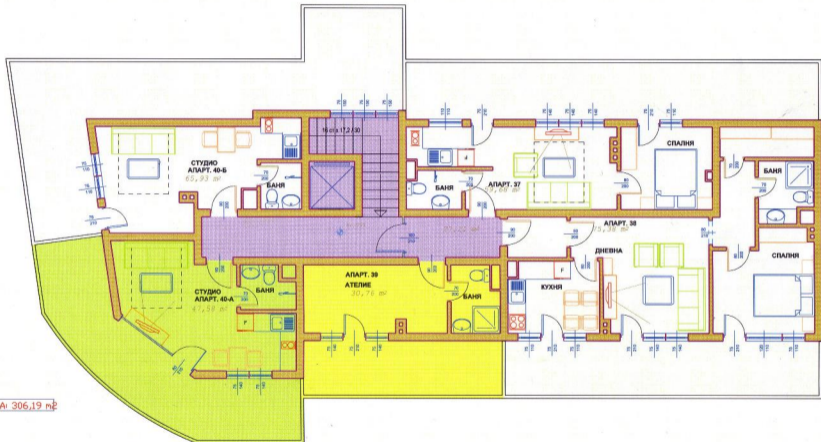
РАЗПРЕДЕЛЕНИЕ И ТЕХНОЛОГИЧНО ОБЗАВЕЖДАНЕ НА ВТОРИ ТЕРАСОВИДЕН ЖИЛИЩЕН ЕТАЖ М 1:50
