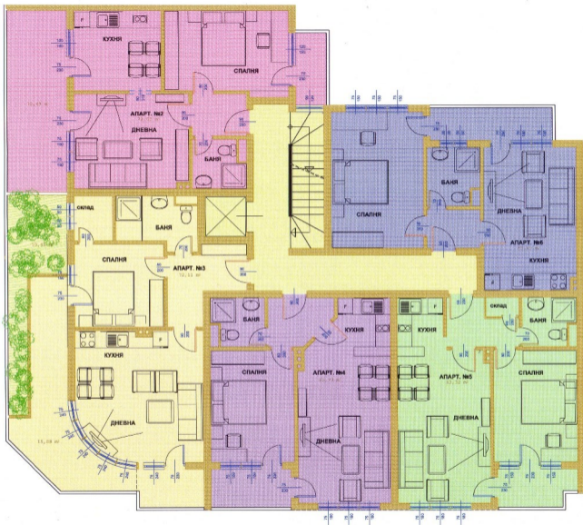
РАЗПРЕДЕЛЕНИЕ И ТЕХНОЛОГИЧНО ОБЗАВЕЖДАНЕ НА ВТОРИ ЖИЛИЩЕН ЕТАЖ М 1:50
