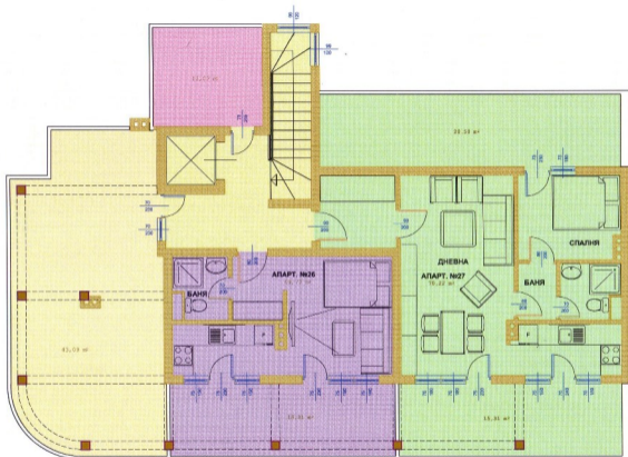
РАЗПРЕДЕЛЕНИЕ И ТЕХНОЛОГИЧНО ОБЗАВЕЖДАНЕ НА ТЕРАСОВИДЕН ЖИЛИЩЕН ЕТАЖ М 1:50
