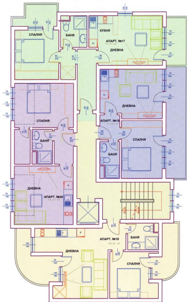
РАЗПРЕДЕЛЕНИЕ И ТЕХНОЛОГИЧНО ОБЗАВЕЖДАНЕ НА ШЕСТИ ЖИЛИЩЕН ЕТАЖ М 1:50
