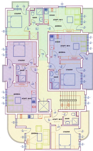
РАЗПРЕДЕЛЕНИЕ И ТЕХНОЛОГИЧНО ОБЗАВЕЖДАНЕ НА ПЕТИ ЖИЛИЩЕН ЕТАЖ М 1:50
