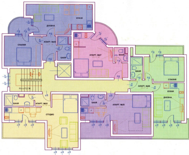
РАЗПРЕДЕЛЕНИЕ И ТЕХНОЛОГИЧНО ОБЗАВЕЖДАНЕ НА ШЕСТИ ЖИЛИЩЕН ЕТАЖ М 1:50
