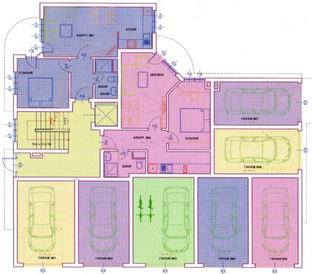
РАЗПРЕДЕЛЕНИЕ И ТЕХНОЛОГИЧНО ОБЗАВЕЖДАНЕ НА ПЪРВИ ПРИЗЕМЕН ЕТАЖ М 1:50
