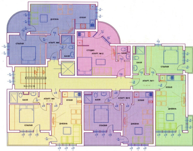
РАЗПРЕДЕЛЕНИЕ И ТЕХНОЛОГИЧНО ОБЗАВЕЖДАНЕ НА ТРЕТИ ЖИЛИЩЕН ЕТАЖ М 1:50
