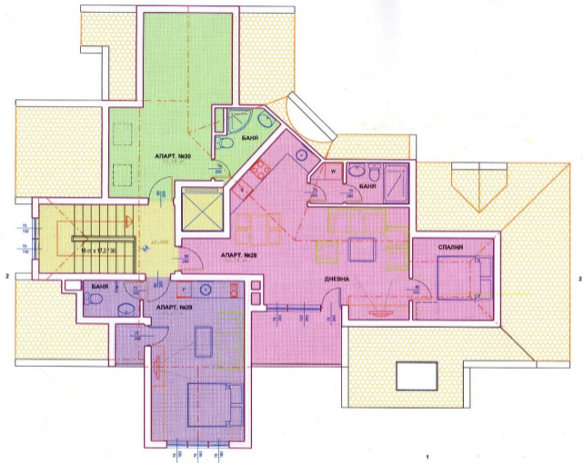
РАЗПРЕДЕЛЕНИЕ И ТЕХНОЛОГИЧНО ОБЗАВЕЖДАНЕ НА СЕДМИ ЖИЛИЩЕН ЕТАЖ М 1:50
