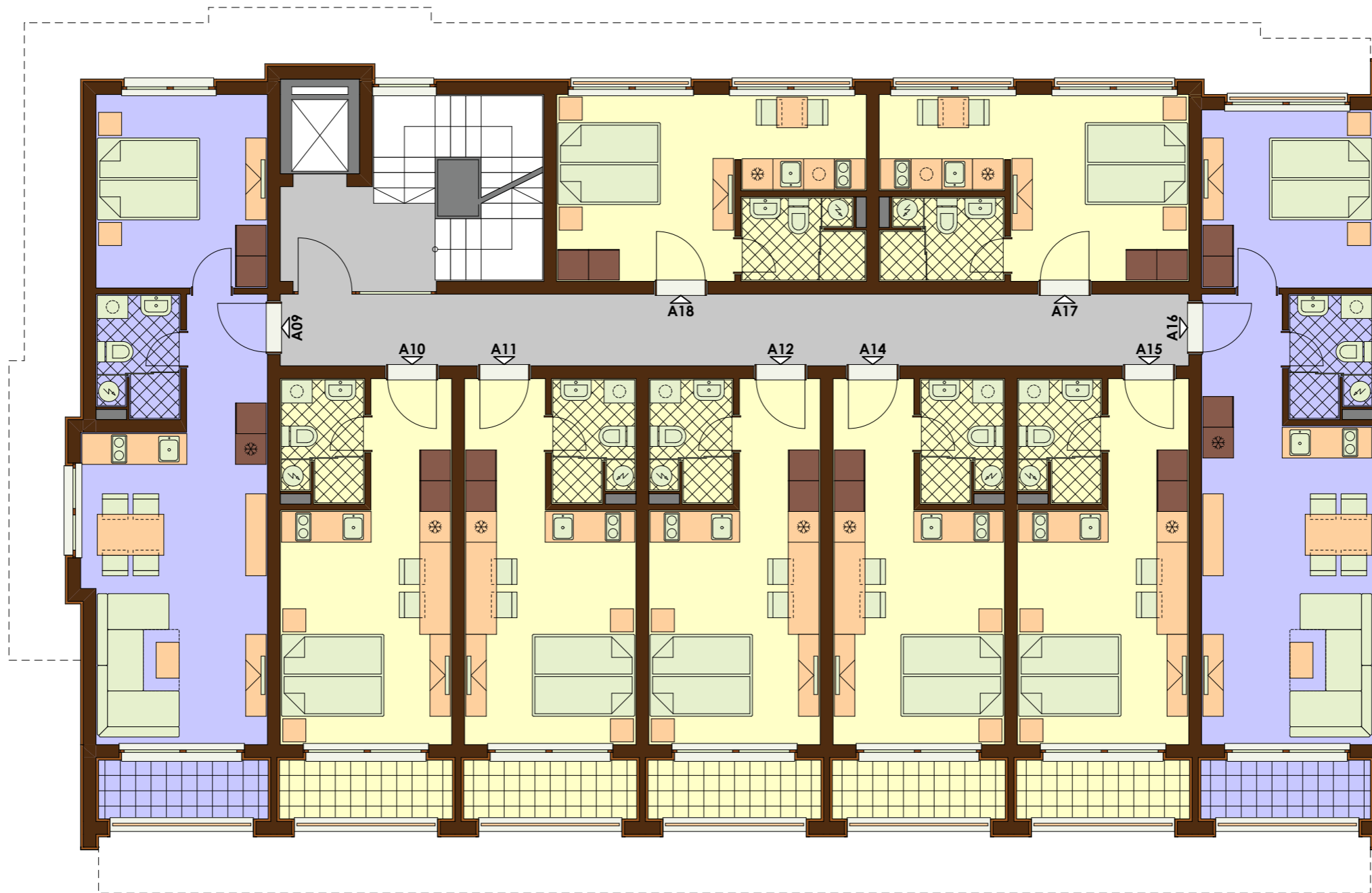
РАЗПРЕДЕЛЕНИЕ ПЪРВИ ЕТАЖ
